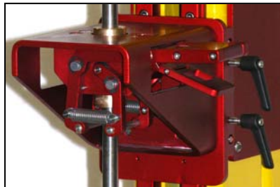
手动重物释放安全装置
