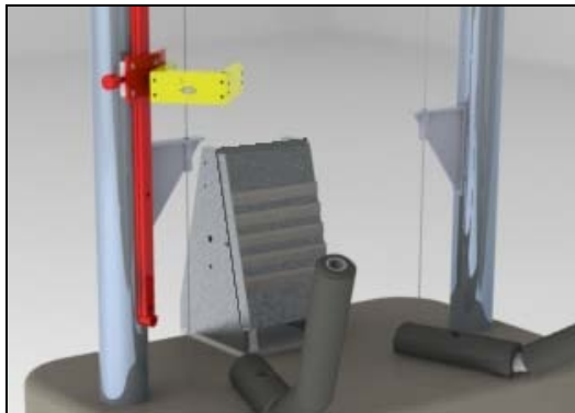
配置测力传感器的砧座，用于测量切向力
