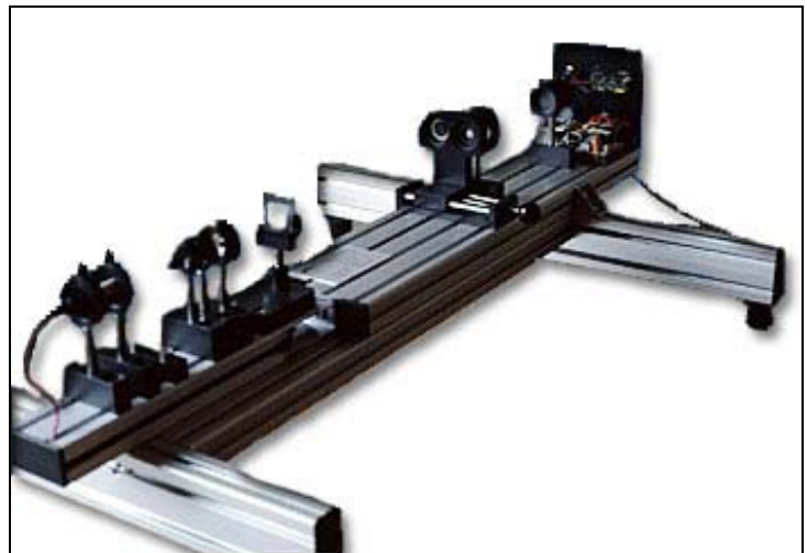
光漫射性能测试台。
