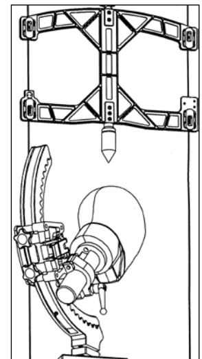
穿刺测试示意图。
