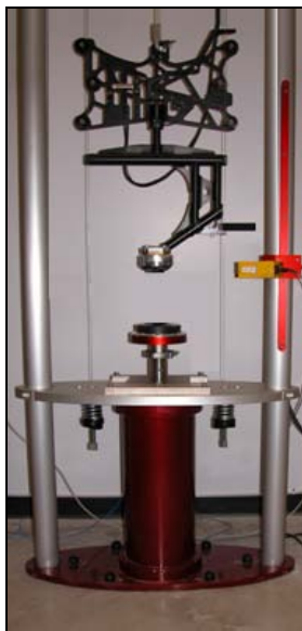
双轨碰撞测试机
