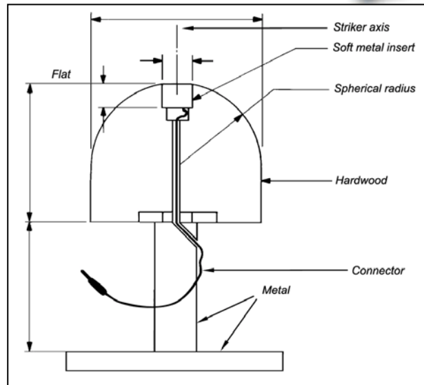
穿刺头模内部结构图.
