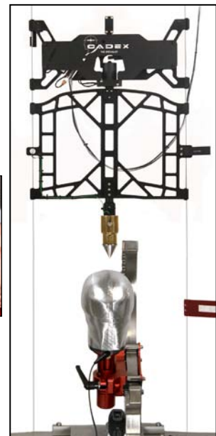
穿刺测试装置示意图
