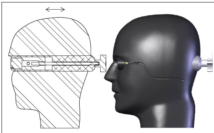
传感器深度调节装置
