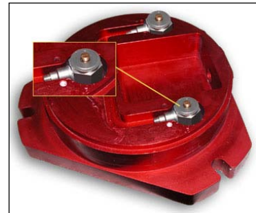
内部视图: 三个等距分布的力传感器 可以达到更高的测量精度。
